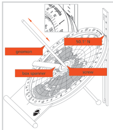
Fig. 6: Setting the latitude
