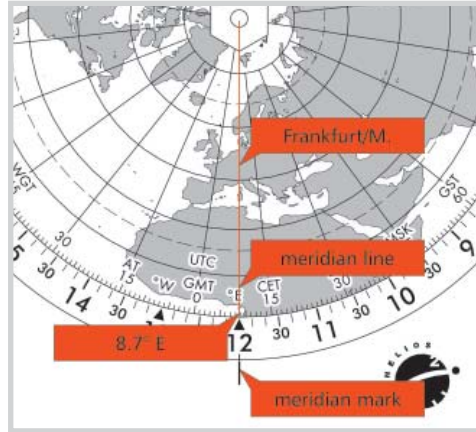
Fig. 5: Setting the longitude
